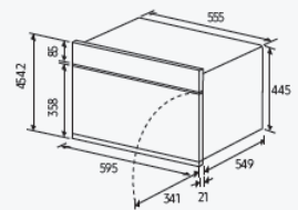
2. 가구장 사이즈
