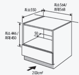
2. 가구장 사이즈
